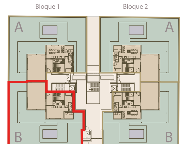
Bloque 1 - bajo B Planta baja
