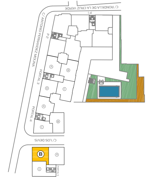
( 2 DORMITORIOS ) PORTAL Nº 5 - PLANTA TIPO ( PLANTAS PRIMERA, SEGUNDA y TERCERA ) VIVIENDA - B
